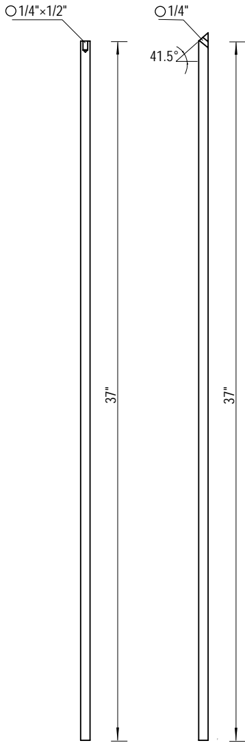
Art.4026 ■ 1/2"×37"
