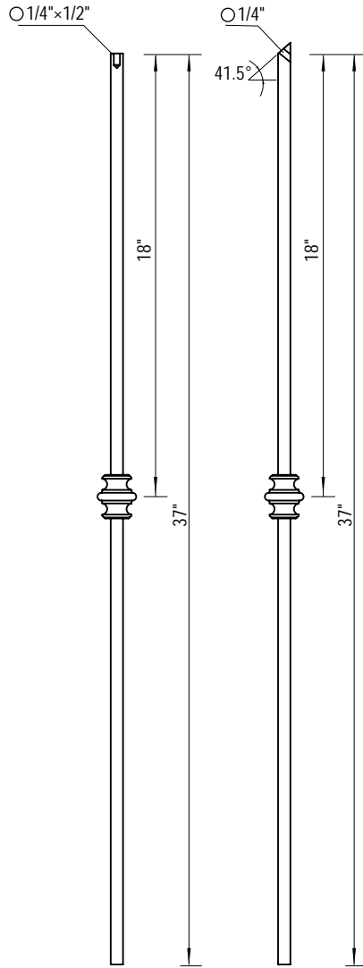
Art.4028 ■ 1/2"×37"
