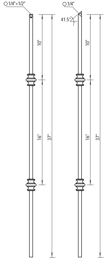
Art.4030 ■ 1/2"×37"
